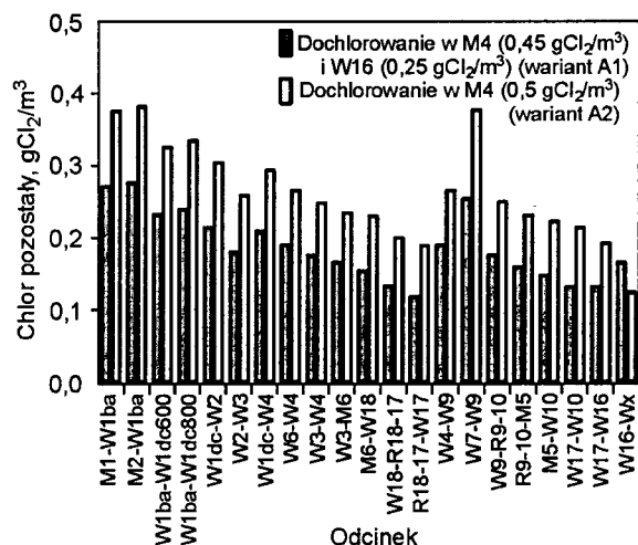
Rys. 9. Porównanie średniej zawartości chloru pozostałego w wodzie w odcinkach zasilanych ze stacji A przy poborze minimalnym i dochlorowaniu w węzłach M4 i W16 (wariant A1) oraz M4 (wariant A2)
