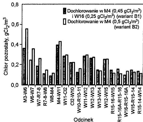
Rys. 10. Porównanie średniej zawartości chloru pozostałego w wodzie w odcinkach zasilanych wodą ze stacji B przy poborze minimalnym i dochlorowaniu w węzłach M4 i W16 (wariant B1) oraz M4 (wariant B2)
